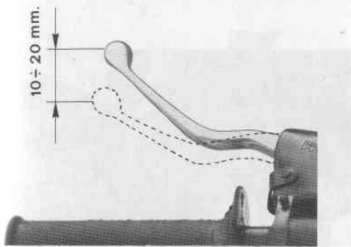
Fig. 15a - Gioco leva frizione
