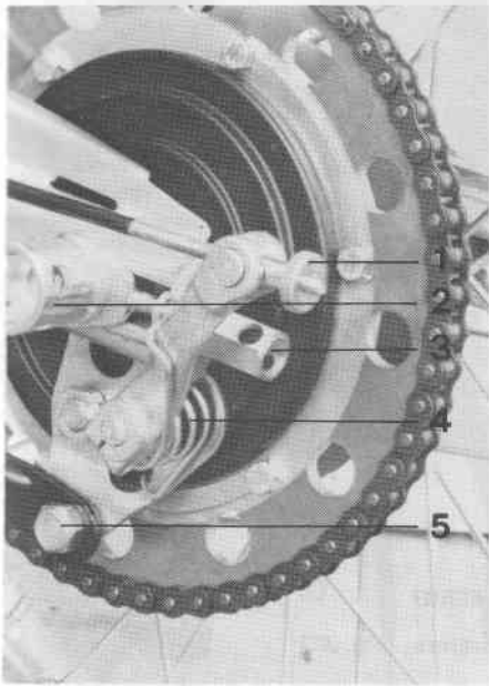
Fig. 39 - Mozzo posteriore
