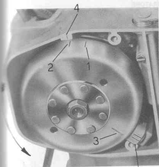
Fig. 34 - Volano DANSI
