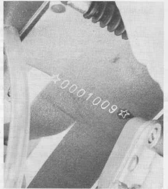
Fig. 4 - Numero Motore
