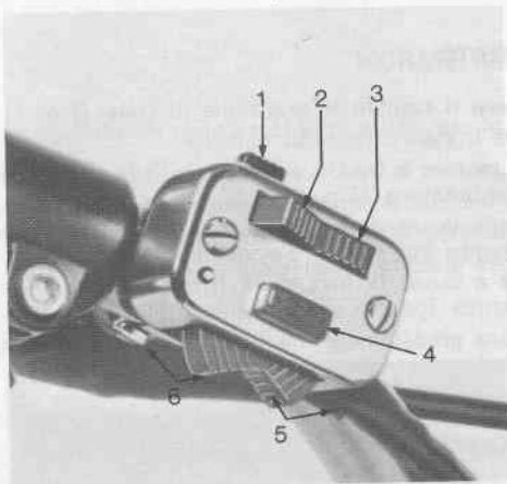
Fig. 5 - Deviatore luci
