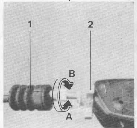
Fig. 22 - Registro leva freno ant.
