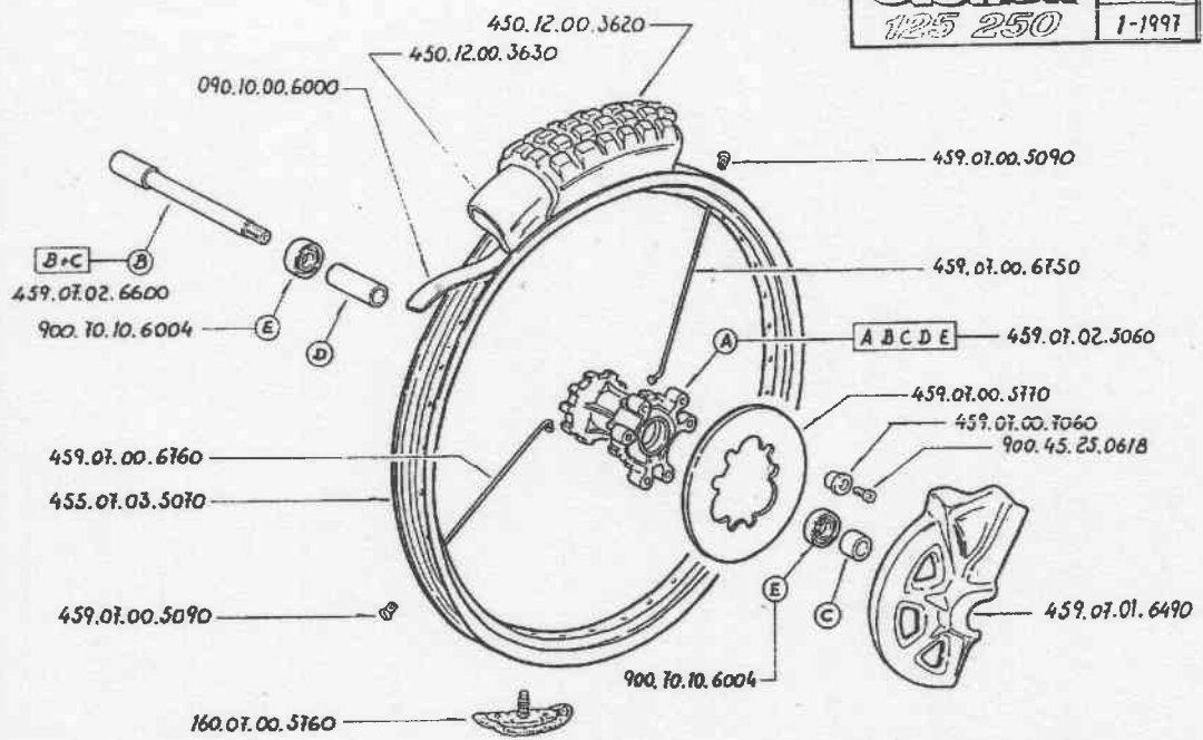
459.07.02.5000 Ruota ant. completa Roue avant complète Front wheel complete Vorderrad Komplett
