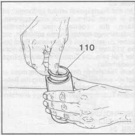
FIG. 25 Sfilare lo scodellino inferiore (110) dal polmone (non utilizzare per questa operazione punte o lame che potrebbero danneggiare il polmone) e rimuovere il polmone (50) dal serbatoio (75). Sostituire il polmone se risulta danneggiato.
