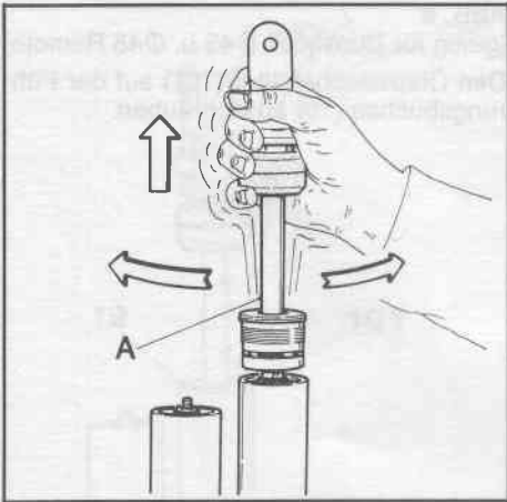
FIG. 8 Estrarre il gruppo asta completo (A) compiendo dei brevi movimenti laterali, come indicato dalle frecce di figura.
