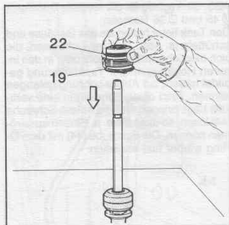
FIG. 32 Rimontare tutti i componenti del gruppo boccola facendo le operazioni in modo inverso allo smontaggio; sostituire l'anello OR (22) con uno nuovo.
