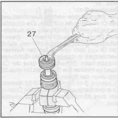
FIG. 33 Inserire tutti i componenti il gruppo ammortizzante fisso di compressione e il gruppo pistone (26); se risultano usurati sostituire i segmenti (25). Con l'asta serrata in mezzo alle ganasce di alluminio, serrare il dado (27) sul pistone con una chiave dinamometrica alla coppia di 7 kgm.
