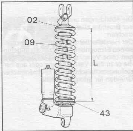
FIG. 1 Prima di eseguire qualsiasi operazione di smontaggio, occorre misurare l'altezza «L» della molla (09). Tale quota va rilevata dalla battuta inferiore dell'anello portamolla (02), alla battuta superiore del registro molla (43). Tale quota dovrà essere rispettata dopo ogni rimontaggio.
