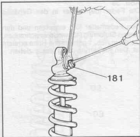
FIG. 40 Inserire il pomello di registro (181) facendo attenzione all'accoppiamento con la vite senza fine precedentemente montata. Avvitare la parte inferiore del registro con una chiave esagonale di 19 mm, mantenendo fermo il pomello di registro con un cacciavite. A questo punto l'ammortizzatore è pronto per l'uso previa regolazione dello smorzamento.
