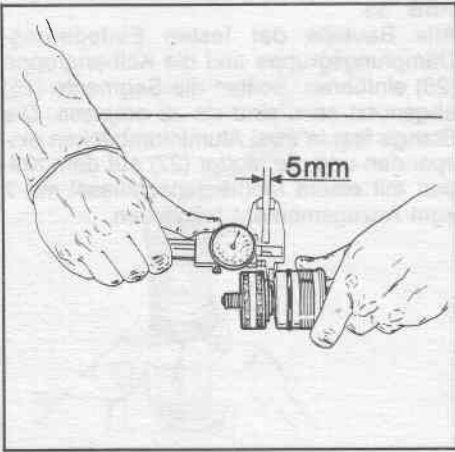
FIG. 35 Distanziare la superficie di fondo della boccia di guida (19) di 5 mm rispetto alla sommità dello scodellino superiore pistone (20). In questo modo risulteranno aperti i fori di circolazione dell'olio all'interno del gruppo asta.
