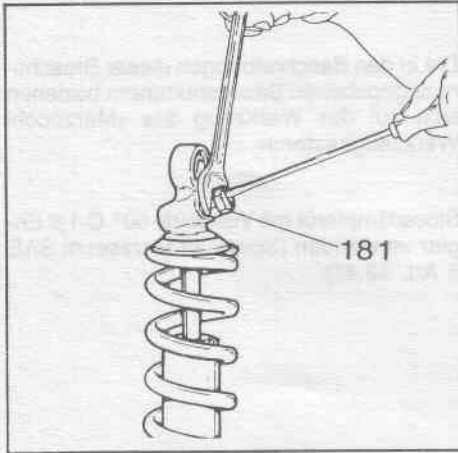
FIG. 2 Portare il pomello di registro (del gruppo valvola 181) nella posizione di minimo smorzamento, posizione «0». Svitare il registro completo utilizzando una chiave esagonale di 19 mm e un cacciavite. Con quest'ultimo mantenere fermo il pomello e contemporaneamente svitare il registro utilizzando la chiave sopraccitata.
