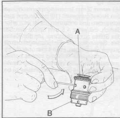
FIG. 20 Appoggiare il gruppo di controllo compressione su di un piano nel modo rappresentato in figura. Con una punta inserita nei fori del cilindretto distanziatore fare leva spingendo sotto alla parte superiore (A); in questo modo si otterrà la separazione del gruppo. Se l'operazione è stata eseguita correttamente avremo tutto il gruppo lamellare e il puntale inserito nella parte (B).
