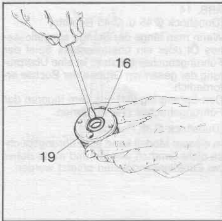
FIG. 16 (valido per Duoshock \varnothing 45 e \varnothing 45 Remoto) Sfilare l'anello raschiatore (16) dal lato opposto della boccia di guida (19) utilizzando un cacciavite. Sostituire sempre l'anello raschiatore ad ogni rimontaggio.
