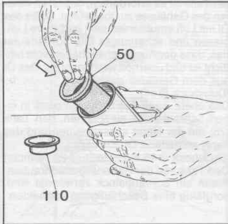
RIMONTAGGIO FIG. 26 Ingrassare tutta la superficie esterna del polmone (50) e dello scodellino (110). Inserire il polmone all'interno del serbatoio portandolo a contatto con l'anello di supporto (111). Inserire poi lo scodellino all'interno del polmone e ingrassare la faccia che andrà a far tenuta sull'anello OR (109).
