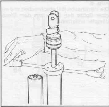
FIG. 7 Posizionare l'occhio superiore dell'ammortizzatore in una morsa e, utilizzando l'apposita chiave (rif. 17-9), per i modelli Duoshock \varnothing 45 e \varnothing 45 Remoto e una chiave esagonale di 40 mm, per il modello \varnothing 38 Remoto, svitare la boccola di guida.
