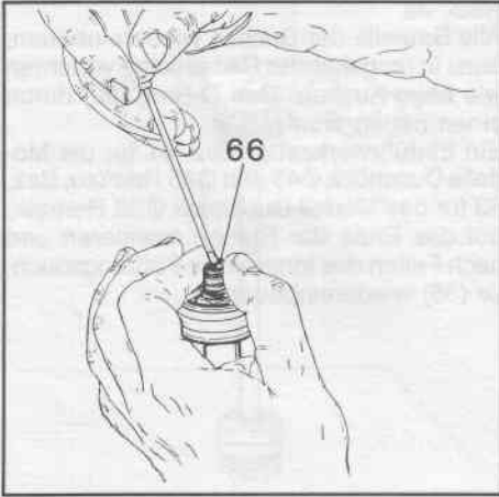
FIG. 34 Inserire sull'estremità del tirante di comando del registro in estensione tutti i componenti nell'ordine di fig. 10. Inserire l'anello di arresto (66).
