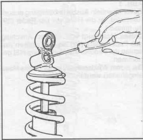
FIG. 3 Smontato il gruppo di comando della regolazione, inserire la punta di un piccolo cacciavite nel foro di accoppiamento della vite senza fine e rimuovere quest'ultima ruotandola in senso antiorario.
