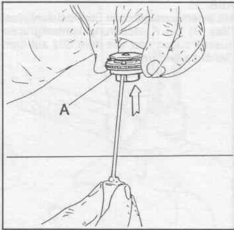
FIG. 21 Operando sulla parte (A) del gruppo di controllo compressione è possibile verificare il comportamento della valvola che controlla il passaggio dell'olio attraverso il gruppo stesso. Inserire un cacciavite sottile nei fori della valvola e, vincendo la forza della molla superiore, sollevare il gruppo di lamelle che chiude il passaggio dell'olio. Controllare che non vi siano particelle che ostruiscano i fori o che impediscano alle lamelle un appoggio perfetto.
