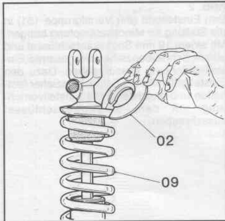
FIG. 4 Allentare con una apposita chiave per ghiera il registro molla inferiore (43 A) e il registro molla superiore (43) fino a che l'anello portamolla (02) risulti libero. Estrarre l'anello portamolla (02) e sfilare la molla (09).
