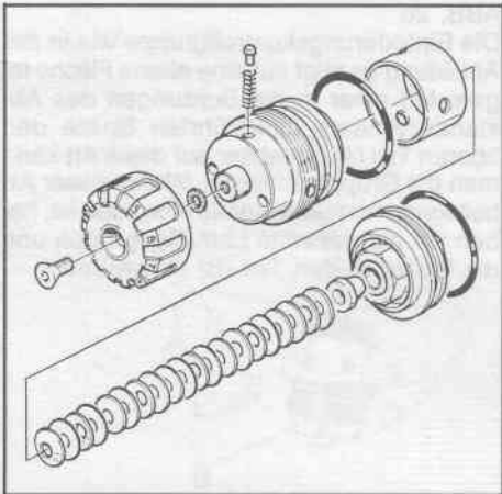
FIG. 22 La figura mostra l'esatto ordine di rimontaggio dei componenti del gruppo di controllo compressione. Fare attenzione al posizionamento delle molle a tazza rispetto alle lamelle. Le molle a tazza devono presentare la parte concava contrapposta e le rondelle devono essere posizionate prima e dopo ogni molla a tazza.
