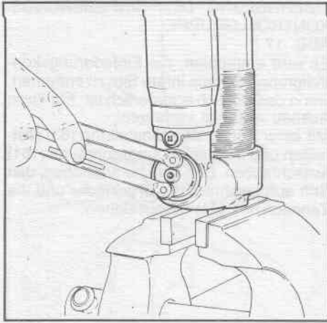
FIG. 19 Con una chiave a compasso (rif. 1) svitare il gruppo di controllo compressione e rimuoverlo dalla sede sulla custodia.
