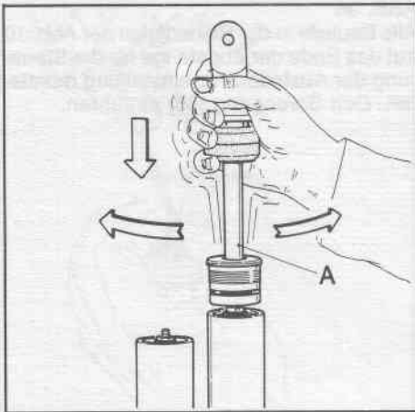
FIG. 36 Inserire il gruppo asta (A) lentamente nella custodia e avvitare la boccia di guida con l'apposita chiave utilizzata nello smontaggio. Duoshock \varnothing 45 e \varnothing 45 Remoto Riavvitare il barilotto (101) con OR (81).
