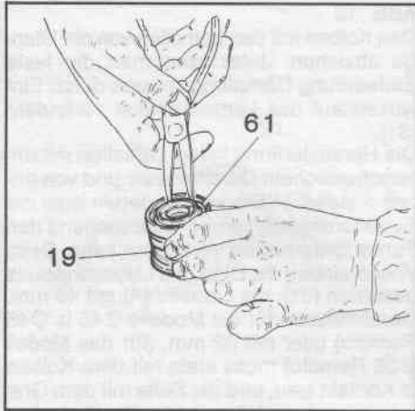
FIG. 14 (Duoshock \varnothing 45 e \varnothing 45 Remoto) Riscontrando perdite d'olio lungo l'asta oppure un eccessivo gioco della boccola di guida è necessario revisionare il gruppo boccola. Rimuovere l'anello di arresto (61) dall'interno della boccola di guida (19).
