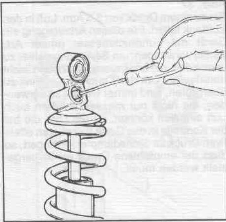
FIG. 39 Reinserire la vite senza fine nell'apposita sede servendosi di un piccolo cacciavite e ruotandola in senso orario.
