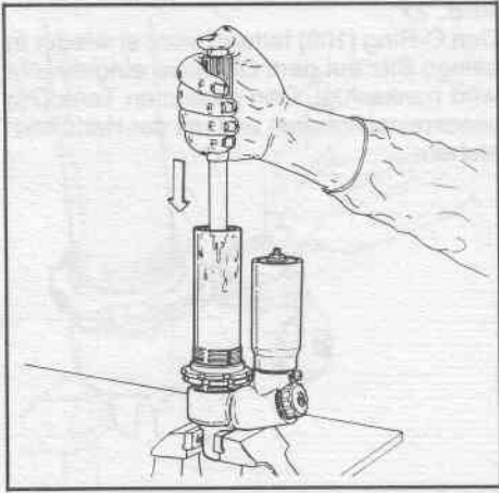
FIG. 29 (valido per il modello Duoshock \varnothing 45 ) Utilizzare per questa operazione l'apposito attrezzo di spurgo (rif. 60) fornito dalla casa costruttrice. Inserire detto attrezzo nella custodia e, premendo il pulsante posto sulla sua sommità, spingerlo lentamente all'inter- no della custodia per circa 20 mm. Rilascia- re il pulsante e svuotare l'olio accumulato sopra all'attrezzo di spurgo.
